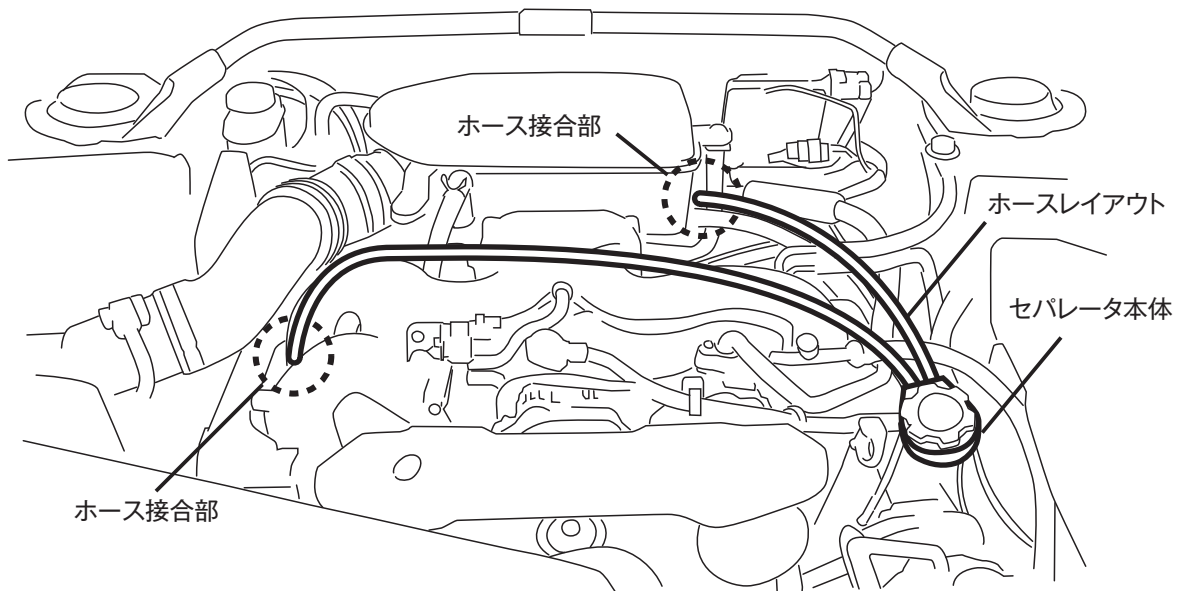
エンジンルームレイアウト図
