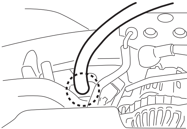
インテークダクト側ホースBを差込みます。 ※ホースを取り回す際、出来るだけ最短距離で 取り回すようにしてください。
