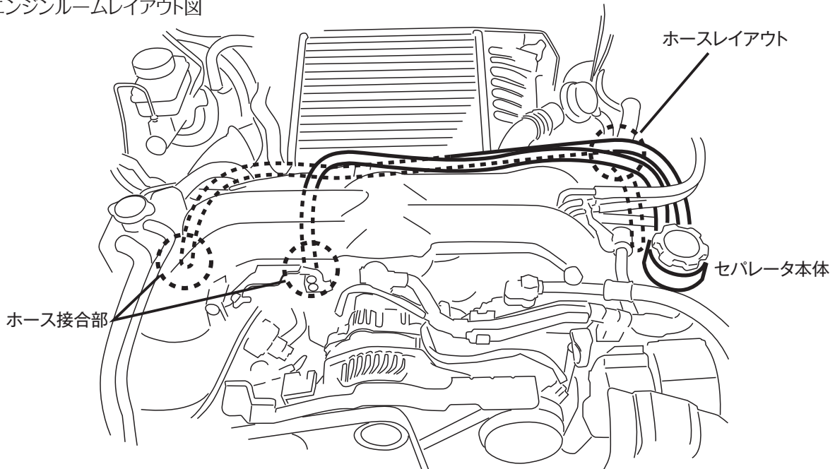
エンジンルームレイアウト図
