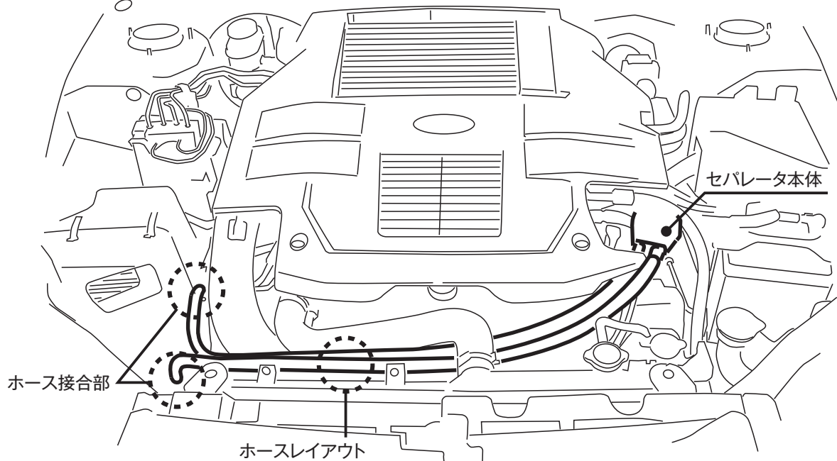
エンジンルームレイアウト図
